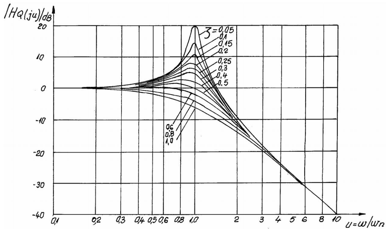
Fig. 1: Caracteristicile de frecventa semilogaritmice exacte pentru un element de intarziere de ordinul 2
